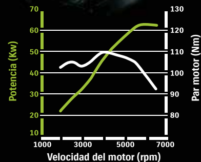
Rendimiento del motor
