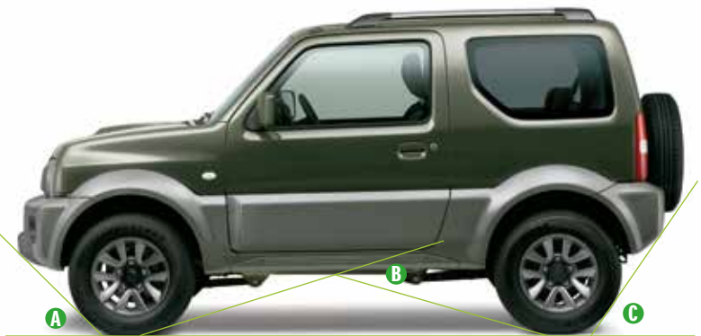
A 34° Ángulo de ataque B 31° Ángulo ventral C 46° Ángulo de salida
