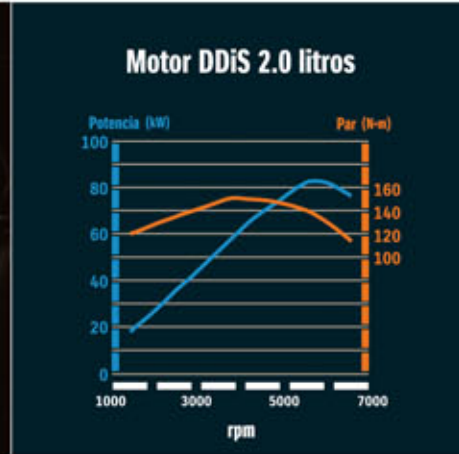
Motor DDiS 2.0 litros
