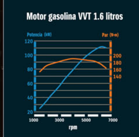
Motor gasolina VVT 1.6 litros
